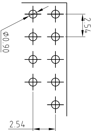
P.C.B LAYOUT
