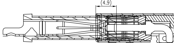
1. NEGATIVE CONTACT PLUG 插入深度 (4.9)
