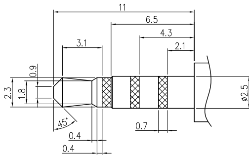
φ2.5 4POLE PLUG(±0.05)
